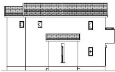
◀南側立面図▶
