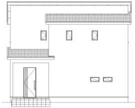
《北側立面図》
