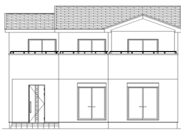
《南側立面図》
