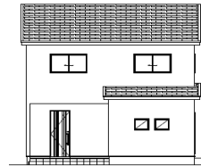
≪北側立面図≫
